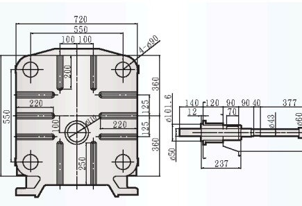
射出關係尺寸圖 INJECTING DIMENSION
