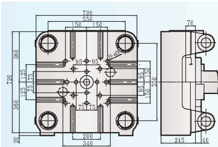
模板押出關係圖 DIE PLATEN DIMENSION
