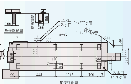
基礎圖 ANCHORING DETAIL
